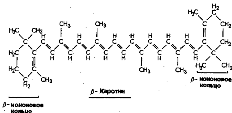
Рис. 12. Структурная формула β-каротина
