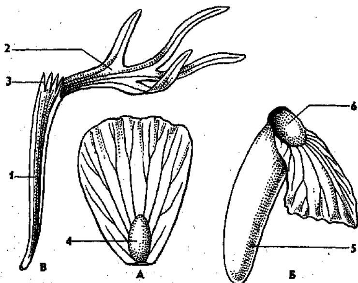
Рис. 91 Примеры видоизменения лепестков (А — сидячий лепесток лютика едкого, образующий в основании нектарную ямку, Б — сидячий лепесток пальцекольника мясокрасного, образующий в основании цилиндрический шпорец, В — ноготковый лепесток коронки кукушкин цвет):
