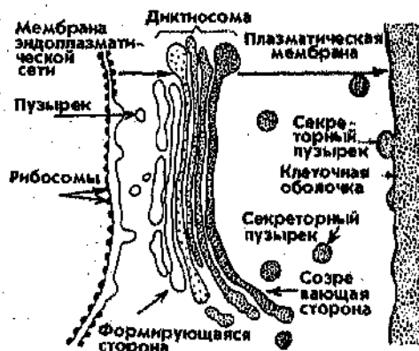
Рис. 6. Взаимодействие и функционирование эндоплазматической сети и аппарата Гольджи (жирной стрелкой показан направленный транспорт синтезируемых веществ)
